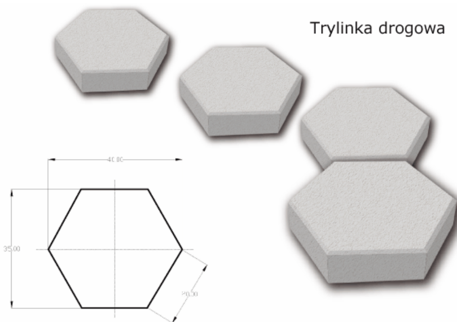
Rys. Trylinka drogowa - wymiary
